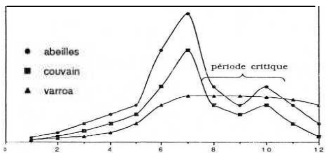
Cycles biologiques d'une colonie d'abeilles et de l'infestation Varroa. Le croisement des courbes indique la période critique (nombre élevé de parasites par larve du couvain).
